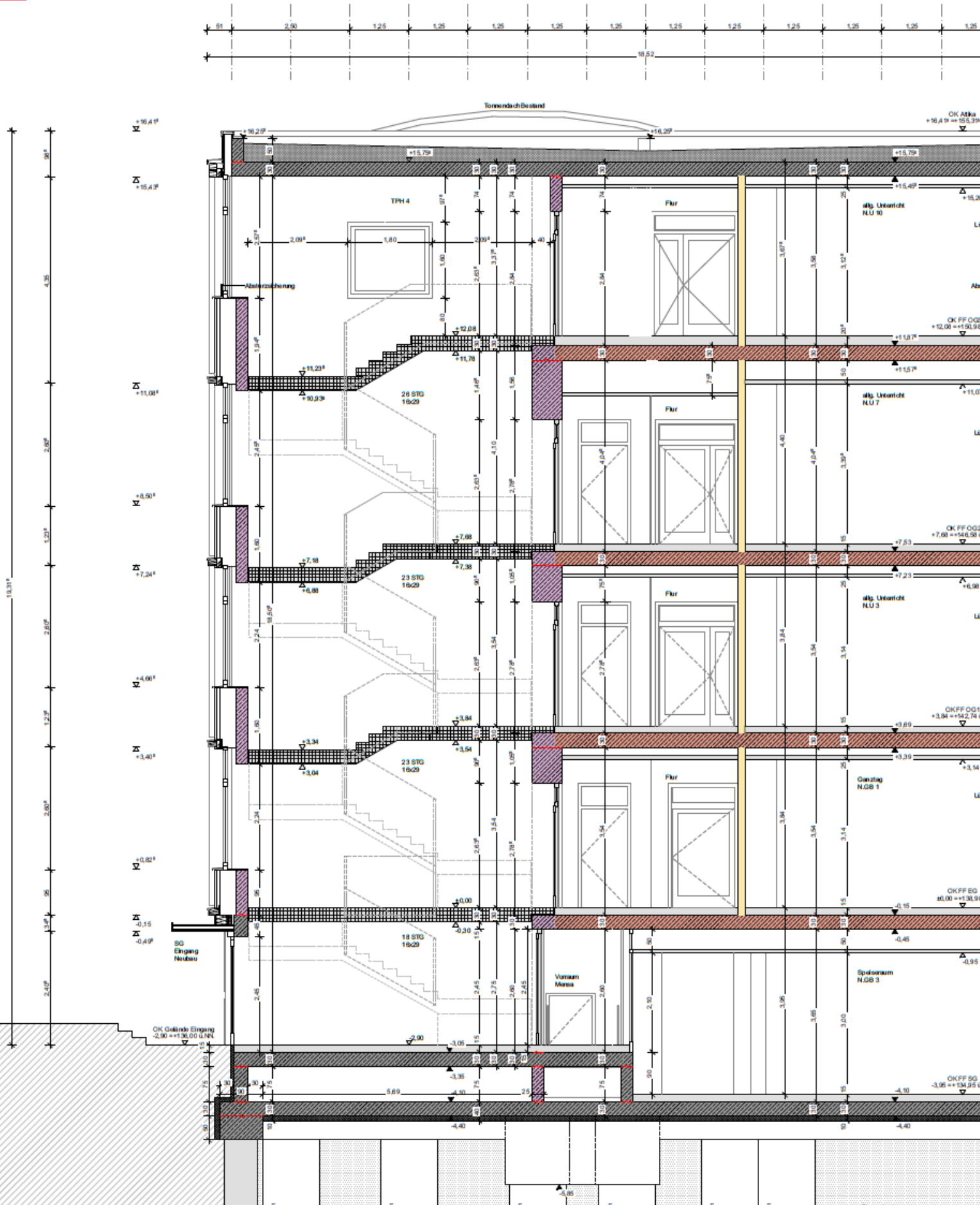
Schnitt C-C
