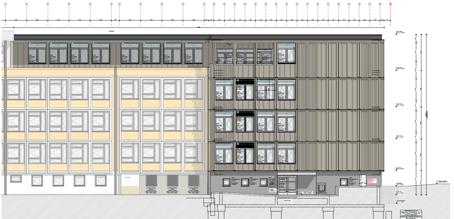
Ansicht Augustinerhof
