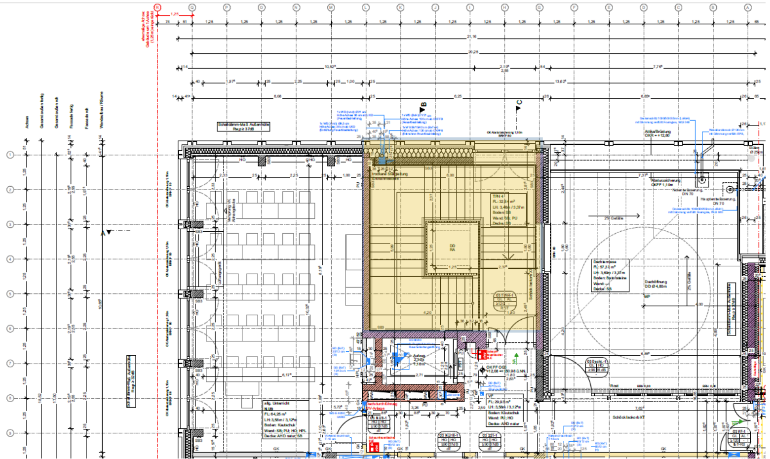
Ausschnitt Grundriss 3.OG
